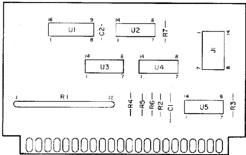
AI2 hp Part No. 03490-66512
